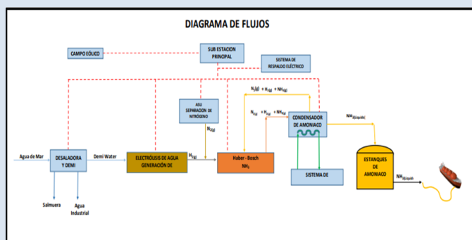
Figura 9. Diagrama de flujo planta amoníaco
